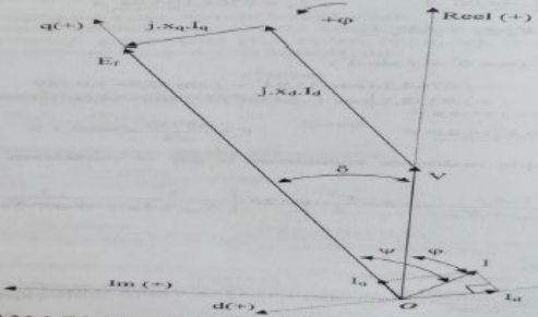
Şekil 34-1 Çukuk kutuplu senkron generatörde vektör diyagramı
